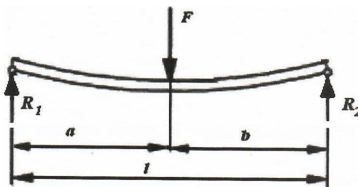
Рисунок 7.2 — Расчетная схема с отброшенными опорами
