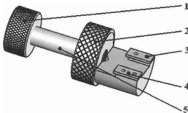
Рисунок 2.13 — Приспособление для плоских образцов.
