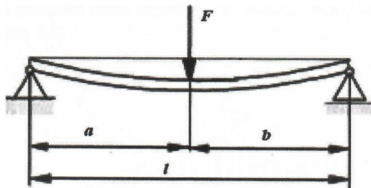
Рисунок 7.1 — Расчетная схема
