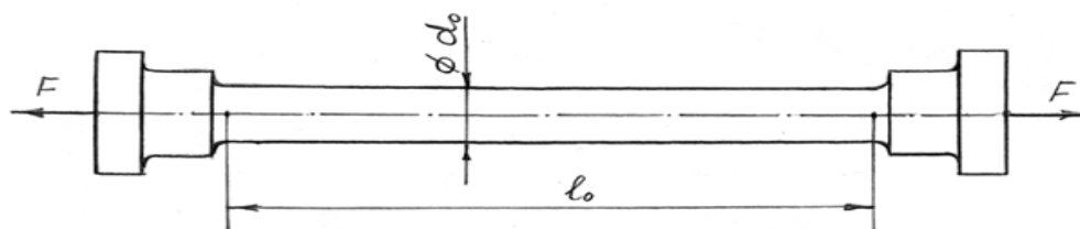
Рисунок 2.4 - Нагружение образца
