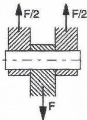
Рисунок 4.2 - Испытание на двойной срез
