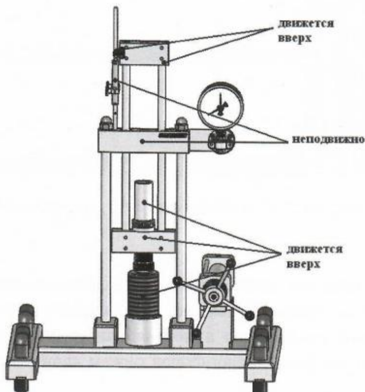
Рисунок 8.10— Направления перемещения частей стенда
