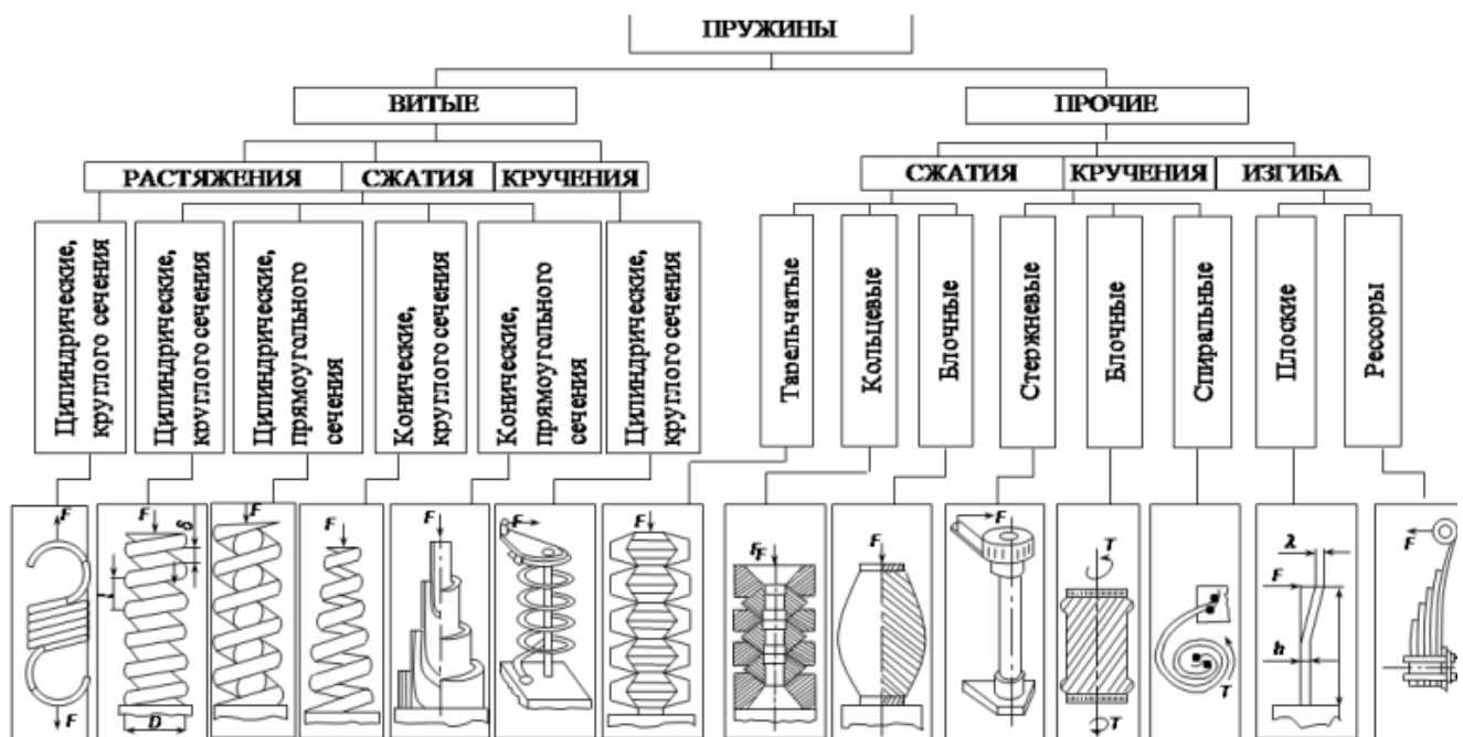
Рисунок 5.1 Классификация пружин
