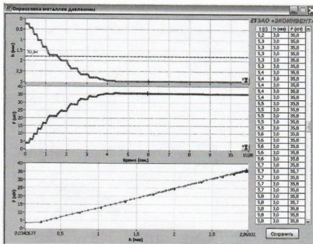
Рисунок 10.13 — Внешний вид программного обеспечения
