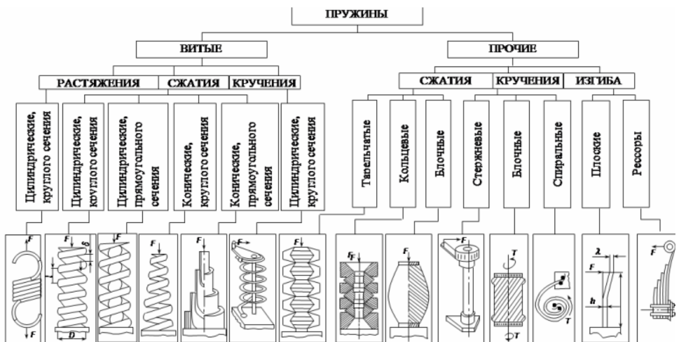
Рисунок 9.1 Классификация пружин
