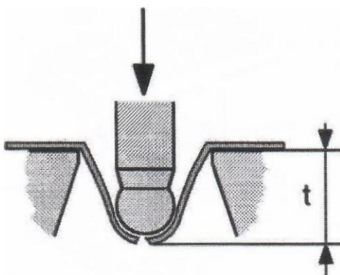
Рисунок 11.2 — Глубокая вытяжка пластины
