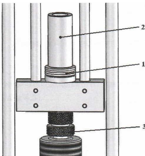
Рисунок 10.6 — Собранная установка
