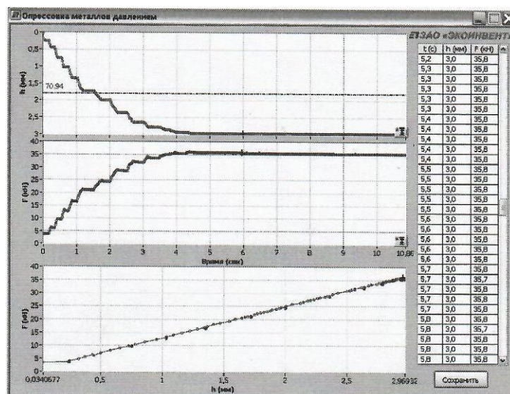
Рисунок 9.11 — Внешний вид программного обеспечения
