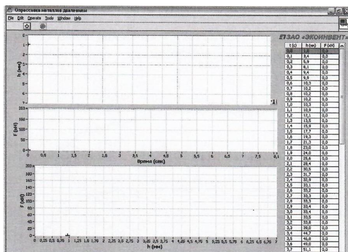
Рисунок 8.5 — Вид программы для работы со стендом Верхнее окно — график смещения во времени Среднее окно — график величины приложенной силы во времени Нижнее окно — график прилагаемой силы в зависимости от смещения образца.
