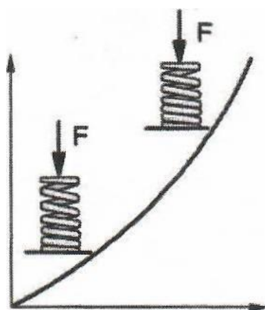
Рисунок 10.2 — Не линейная упругая характеристика цилиндрической пружины
