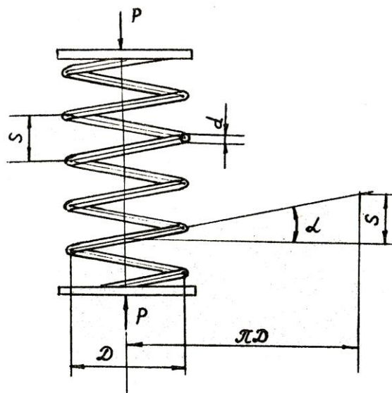
Рисунок 9.2 – Цилиндрическая спиральная пружина
