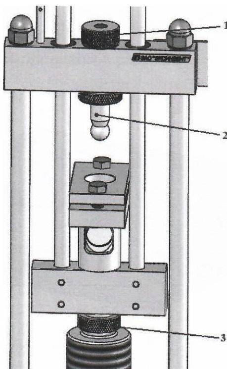
Рисунок 11.5 —Установка в сборе
