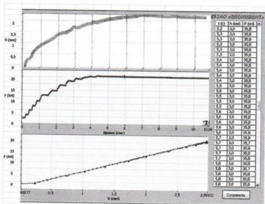
Рисунок 8.7 – Диаграмма нагружений
