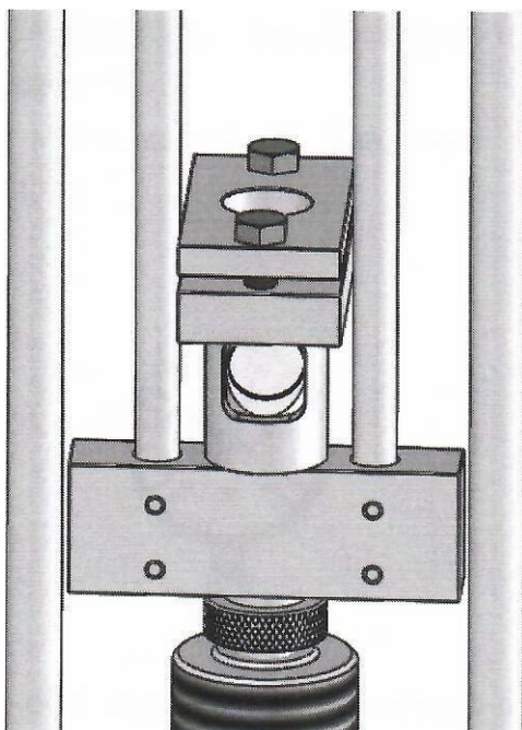
Рисунок 11.4- Установленное приспособление
