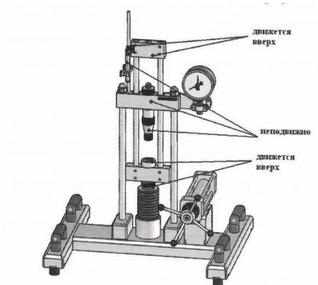
Рисунок 6.5 - Направления перемещения частей стенда
