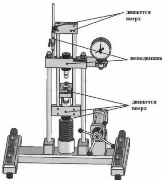
Рисунок 11.8 — Направления перемещения частей станда
