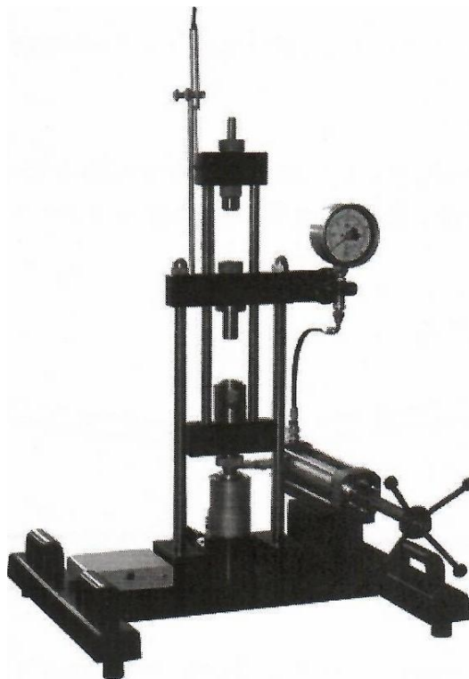
Рисунок 11.1 — Универсальная машина для исследования свойств материала.
