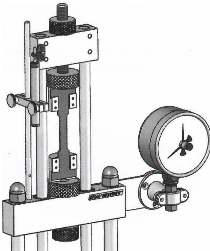
Рисунок 2.14 — Собранный стенд для испытания плоских образцов на растяжение
