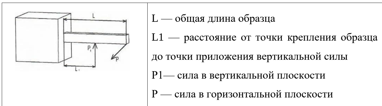
Рисунок 8.2 — Схема нагружения
