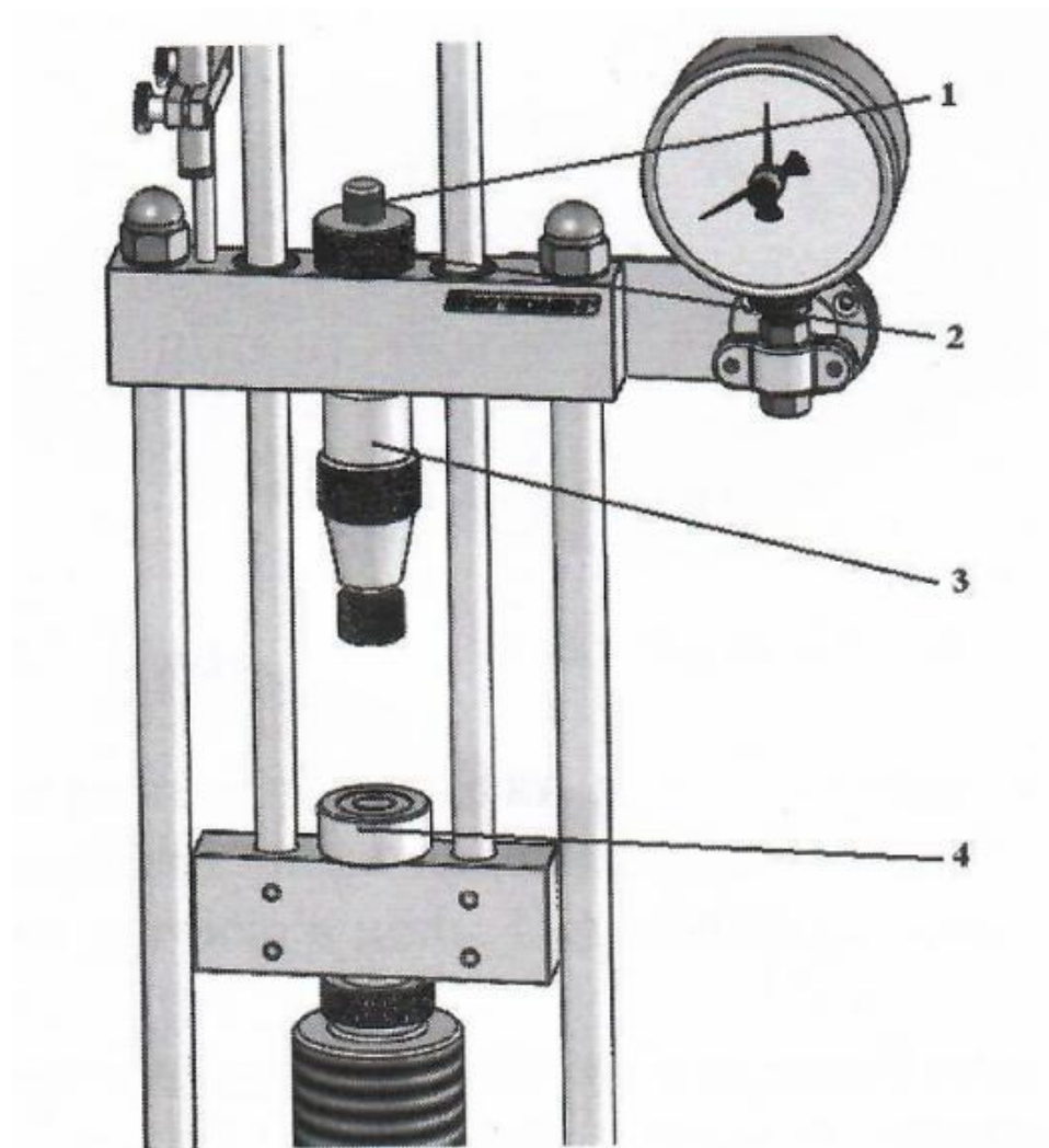
Рисунок 6.3 — Собранный стенд
