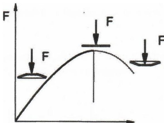
Рисунок 10.4 — График поведения тарельчатых пружин
