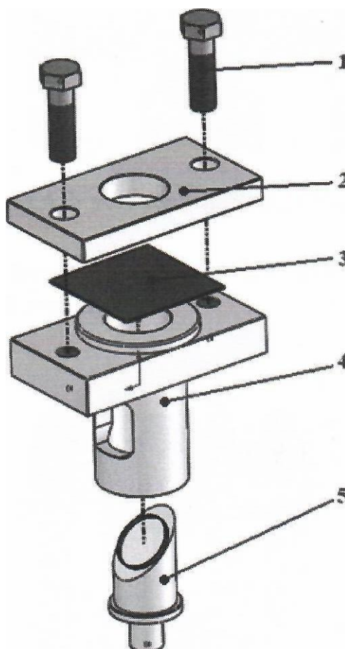
Рисунок 11.3 - Сборка приспособления для испытания
