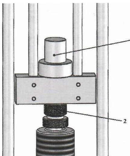
Рисунок 10.5- Собранное приспособление
