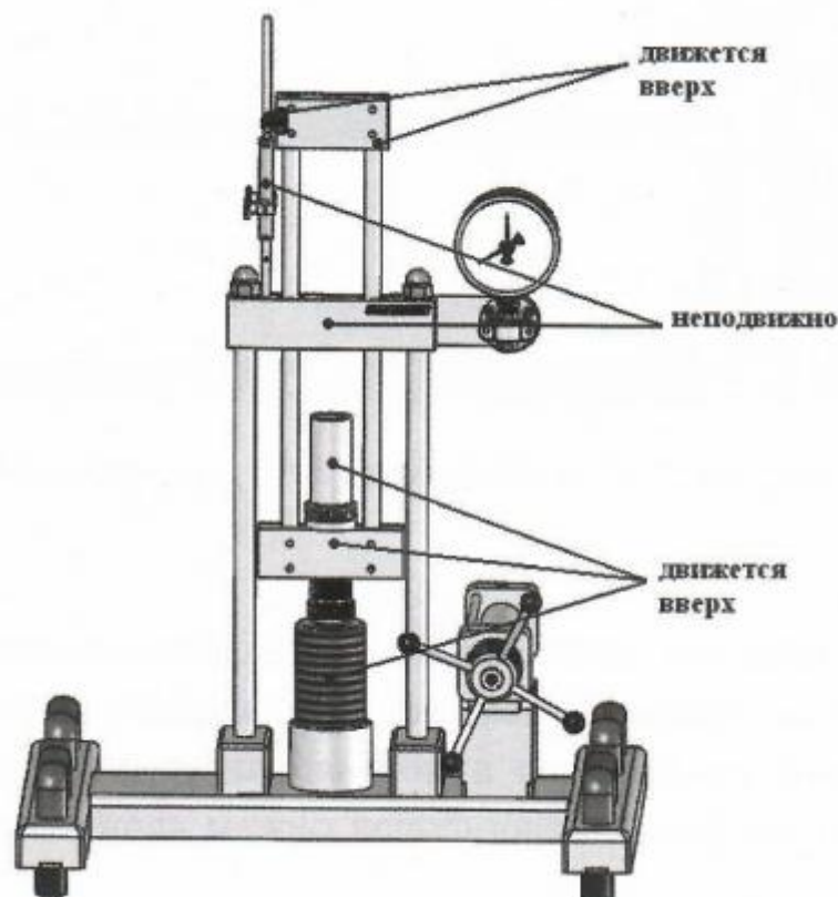
Рисунок 10.11— Направления перемещения частей стенда
