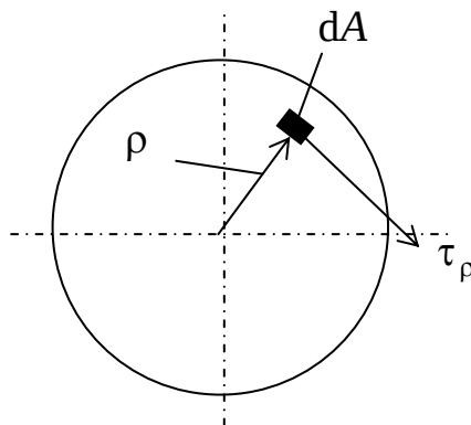
Рис. 1.2. Поперечное сечение вала
