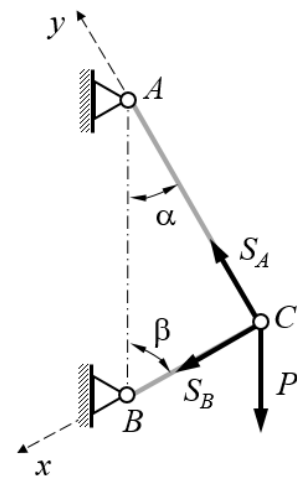
Расчётная схема
