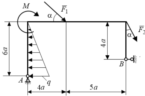
Рис. 1. Исходная схема
