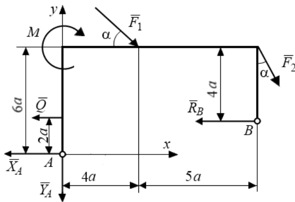
Рис. 2. Расчётная схема
