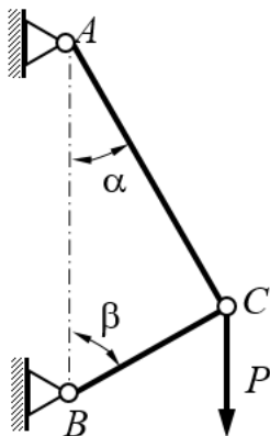
Исходная схема
