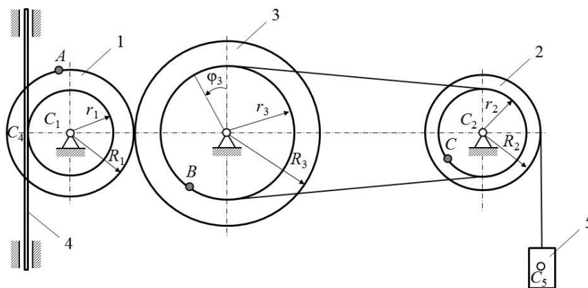
Схема механизма
