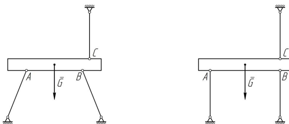
а) статически определимая задача б) статически неопределимая задача
