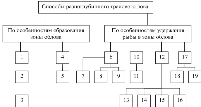
Рис.1.1 Классификационные признаки способов лова разноглубинными травами: 1 - при управлении орудием лова; 2 - путем поступательного перемещения трава; 3 - при постоянной скорости траления; 4 - при управлении объектом лова; 5 - путем использования задерживающих и направляющих функций гидродинамических полей (вихревых шлейфов) траловых досок; 6 - в предустьевом пространстве трава; 7 - путем регулирования скоростью траления; 8 - путем регулирования параметров устья трава; 9 - по принципу наименьшего воздействия световых и гидродинамических полей элементов устья трава; 10 - в передней части трава при обратном выходе из трава; 11 - путем регулирования скорости траления; 12 - в передней части трава при выходе через оболочку трава; 13 - путем регулирования скорости траления; 14 - путем изменения структуры оболочки; 15 - путем изменения сплошности оболочки; 16 - путем регулирования дальности и степени видимости оболочки; 17 - в траловом мешке; 18 - путем регулирования параметров сетного полотна тралового мешка (размера ячеи, диаметра нитевидного материала, относительного рабочего удлинения ячеи); 19 - путем изменения конструкции тралового мешка (показателей покрытия, системы пожил и т.д.).
