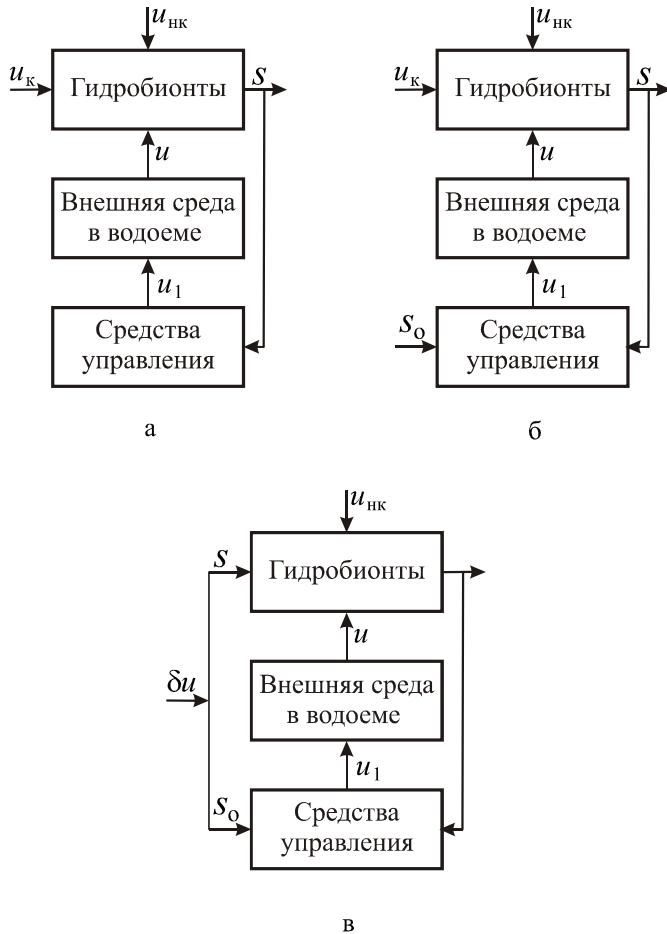
Рис. 2.2. Схемы замкнутых систем управления: а - при управлении по отклонению; б - при программном управлении по отклонению; в - самонастраивающихся
